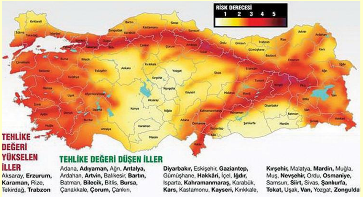
Görsel 96: Türkiye deprem risk haritası
